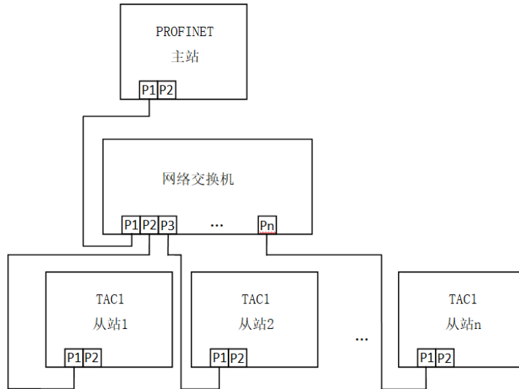
图 9.3 PROFINET 通讯板星型结构图
