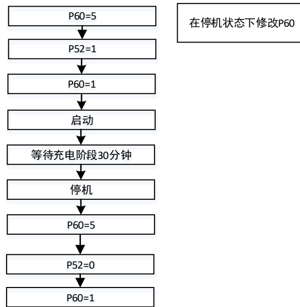
图 10-1 充电步骤
