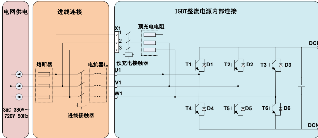
图 2-4 由 IGBT 整流电源组成的整流系统
