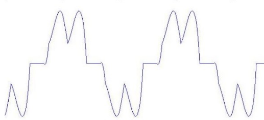
图 2-1 整流状态时交流电流波形
