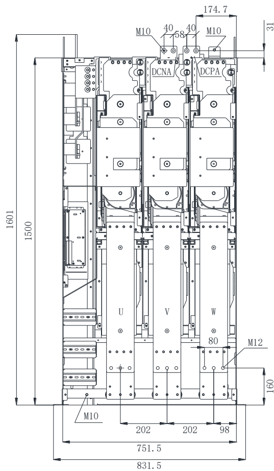
图 3-4 正视图
