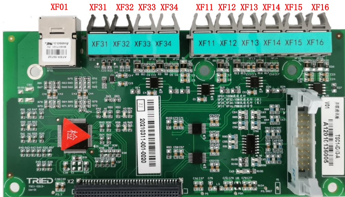
图 4-6 高速通讯板
