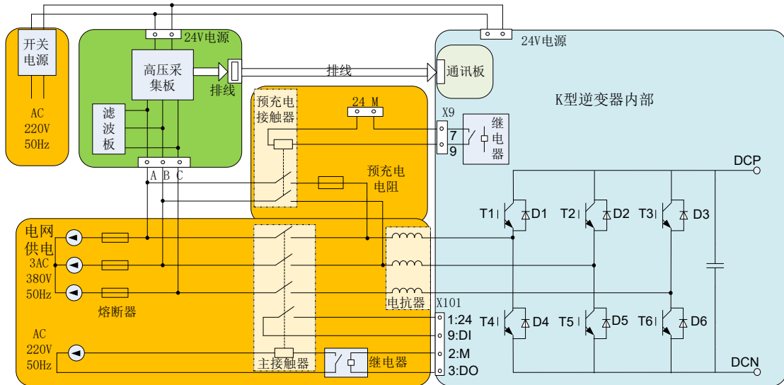
图 2-5 K 型 IGBT 整流电源组成的整流系统
