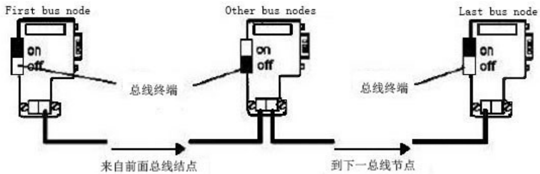
图 8.8 终端电阻的连接示意图
