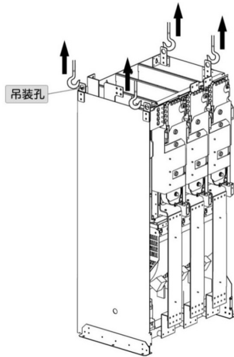
图 3-7 D 型结构吊装图
