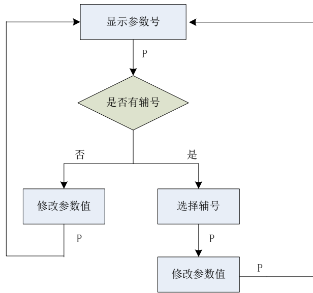
图 5-2 P 参数操作
