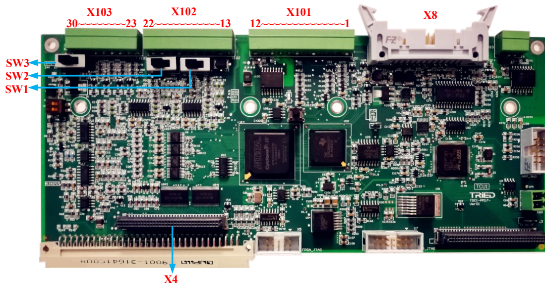
图 4-5 Tried 控制板
