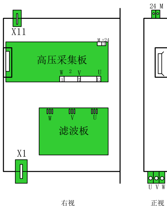
图 2-9 电压检测单元接口图
