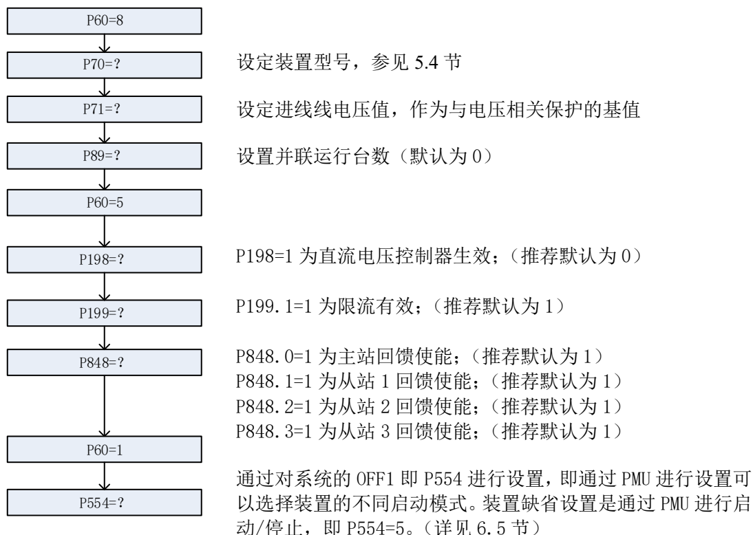
图 5-10 第一次启动设置
