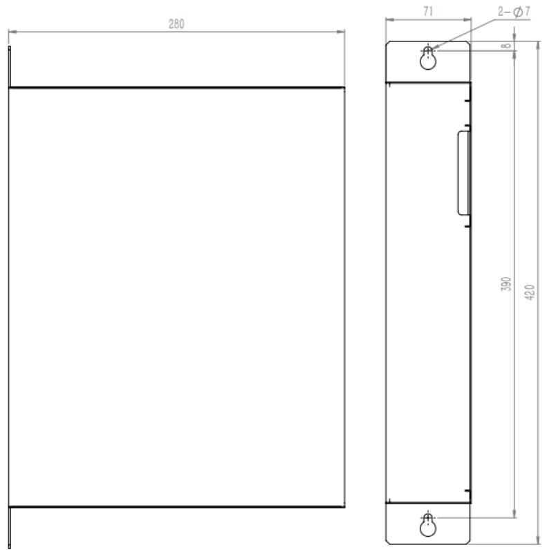
图 2-7 检测单元盒尺寸图
