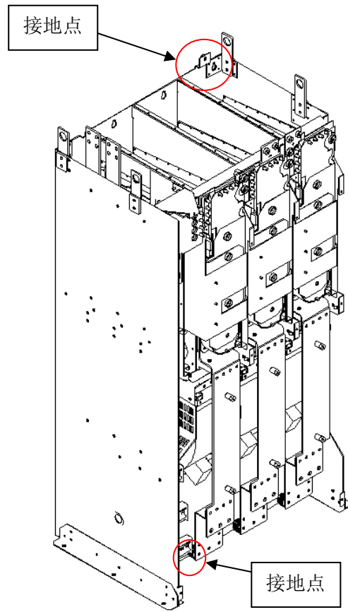
图 4-2 IGBT 整流电源接地位置
