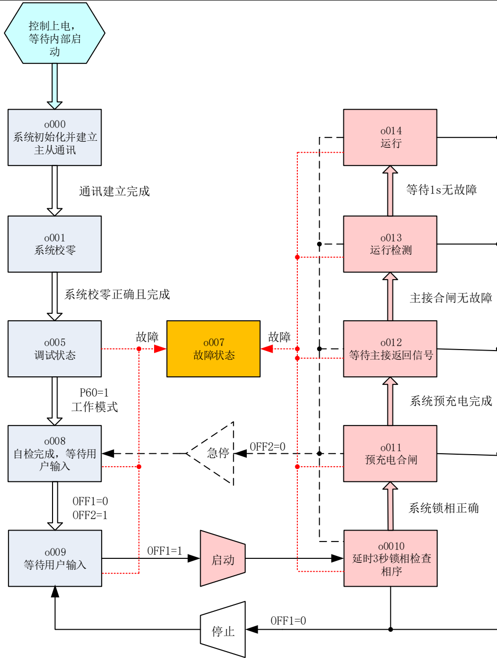
图 6-1 系统启停逻辑图
