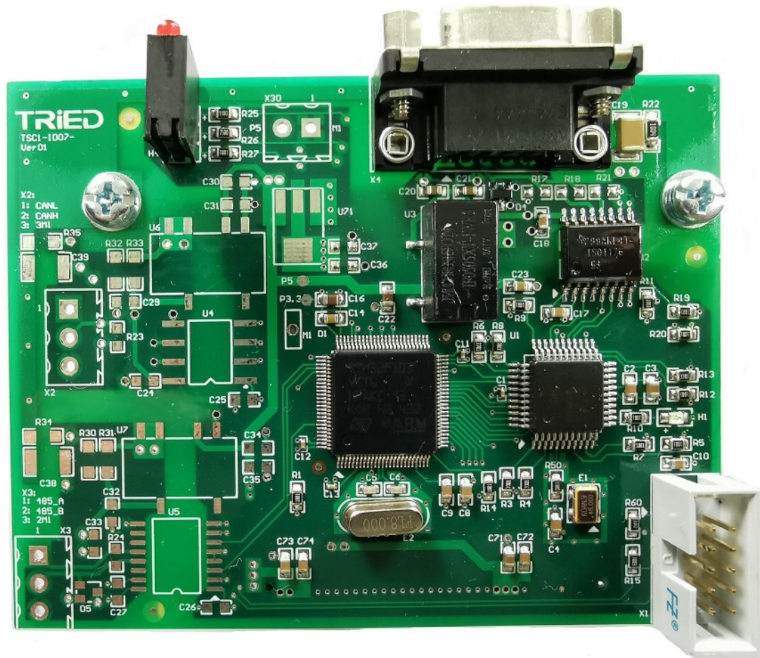
图 8.5A DP 通讯板俯视图
