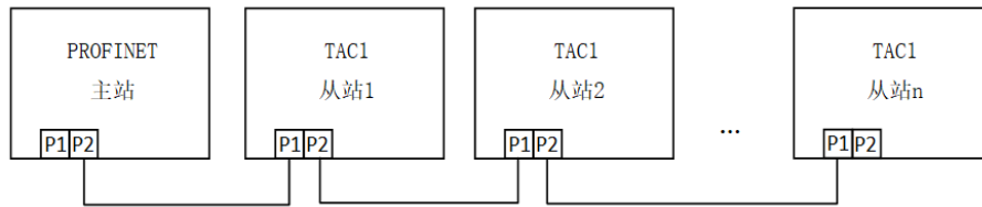
图 9.2 PROFINET 通讯板总线型结构图
