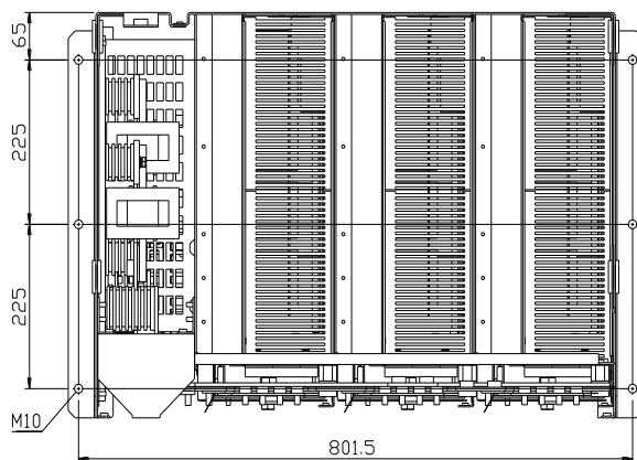
图 3-5 顶视图
