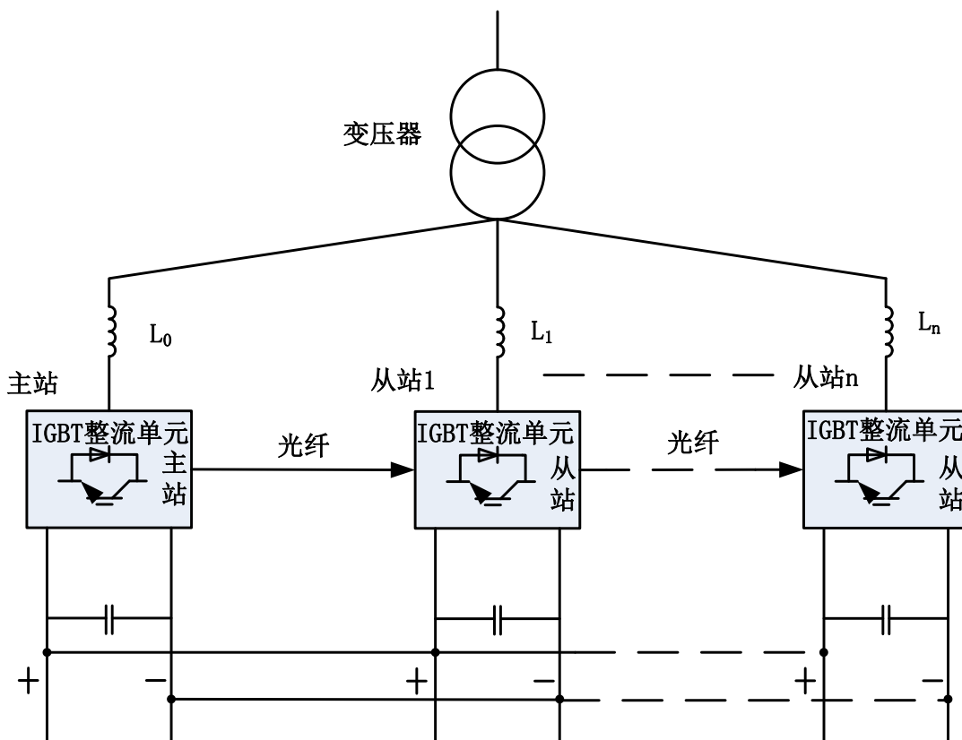
图 2-6 6 脉冲并联方式
