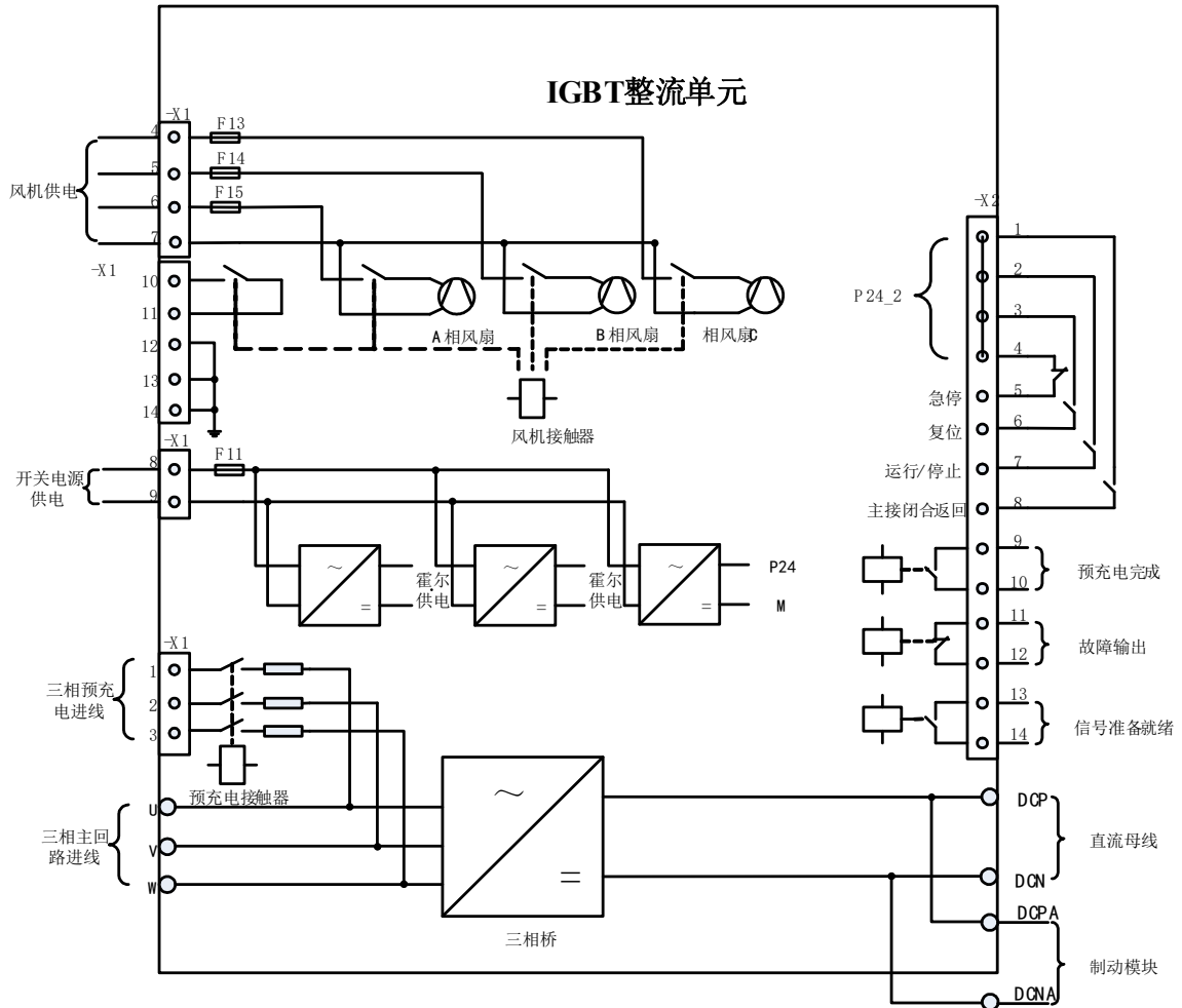
图 4-3 IGBT 整流电源内部结构
