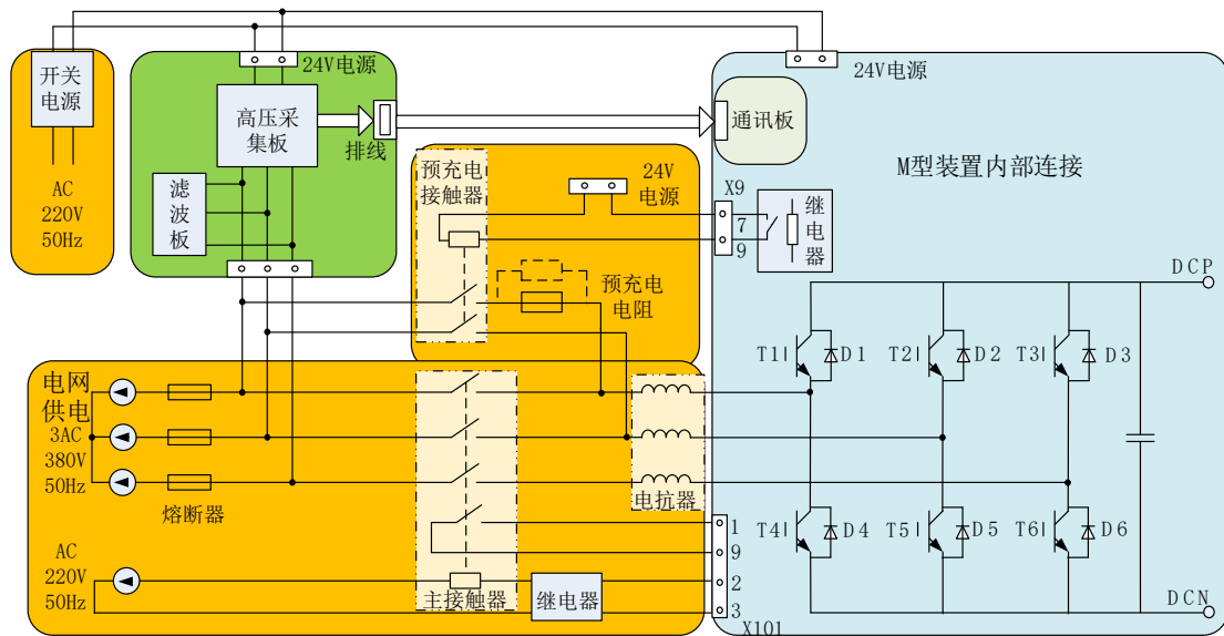
图 2-8 M 型 IGBT 整流电源组成的整流系统
