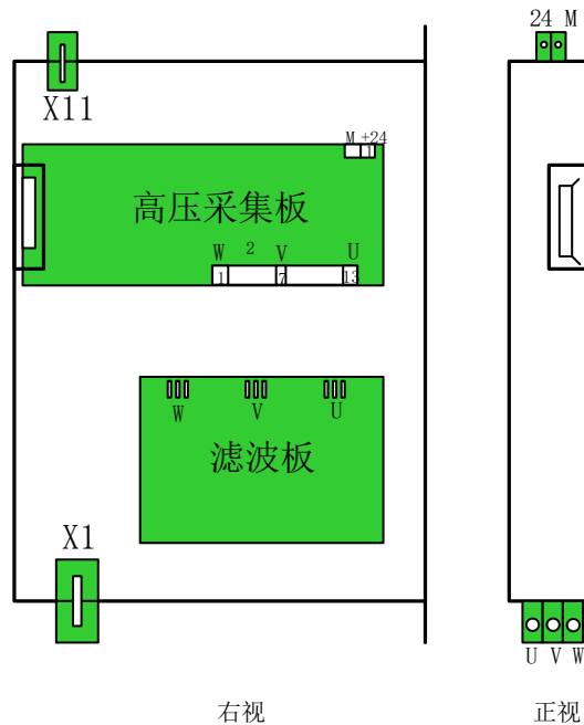
图 2-6 电压检测单元接口图
