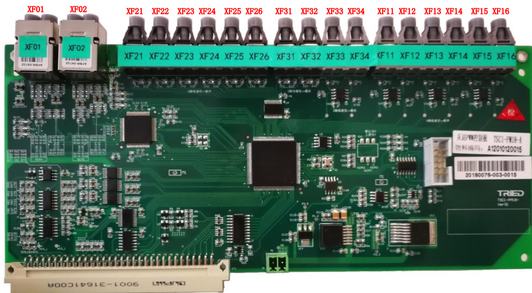
图 4-4 PWM 板
