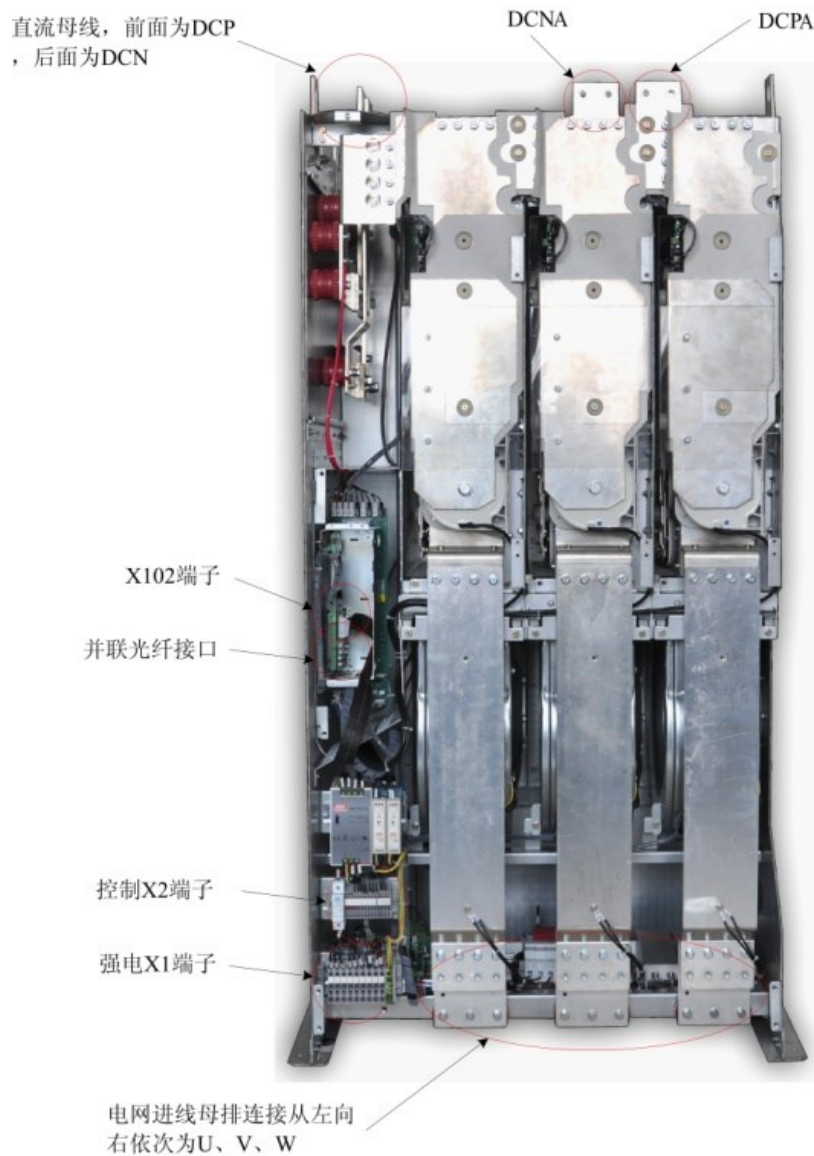
图 4-1 IGBT 整流电源接口位置
