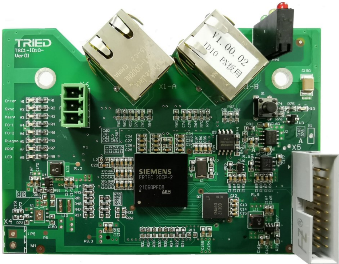
图 9.1A PN 通讯板俯视图
