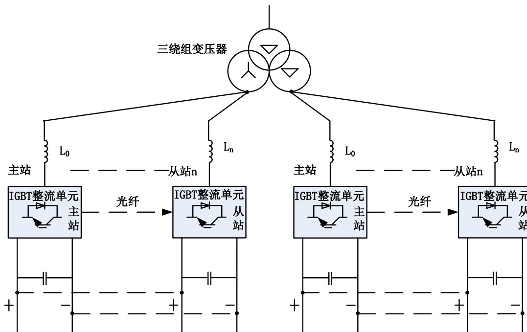
图 2-7 12 脉冲并联方式
