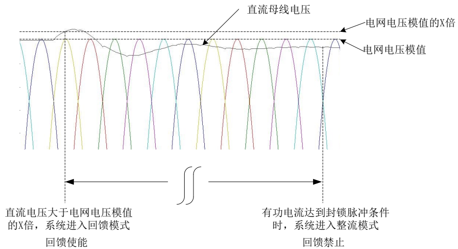
图 7-1 电压控制器脉冲控制示意图
