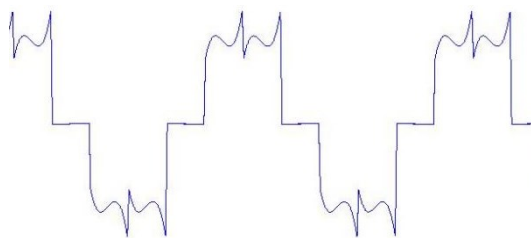
图 2-3 回馈电流波形
