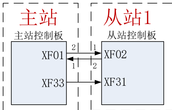
图 4-7 两台 IGBT 整流电源并联光纤连接图
