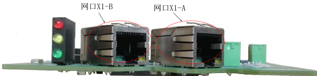
图 9.1B PN 通讯板正视图
