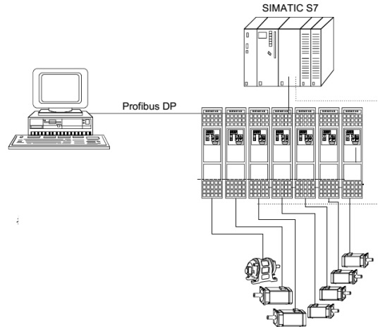
图 8.1 通讯
