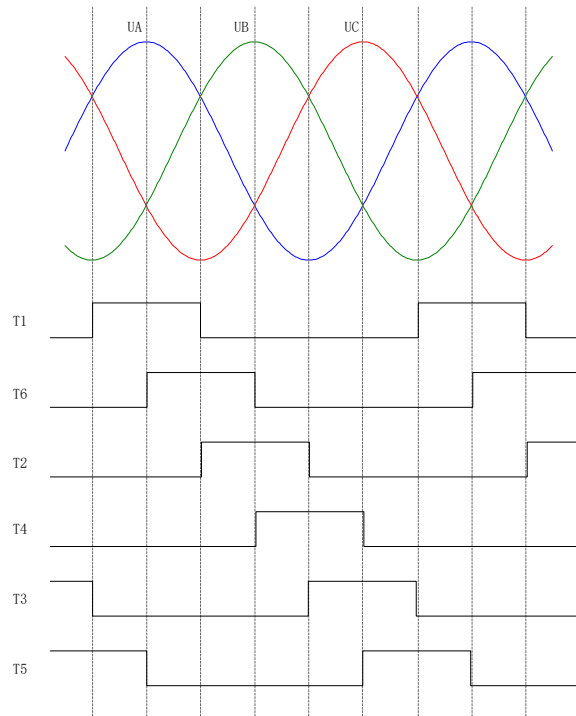
图 2-2 IGBT 导通方式 (参考图 2-4)
